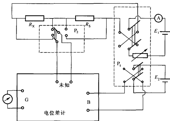
图 D1 电位差计测量电阻原理图
