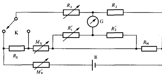
图 B2 四端式电桥置换法测量电桥电阻
