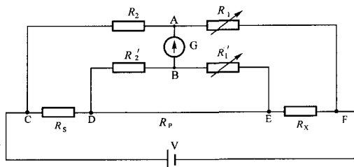
图2 四端式电桥节点位置
