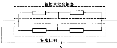
图4 量程变换器整体检定
