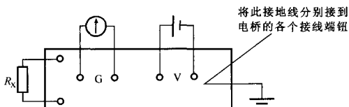
图3 电桥绝缘电阻对整体误差影响试验
