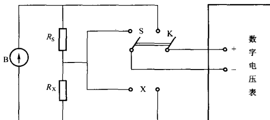
图 C1 恒流源、数字电压表测量电阻原理图
