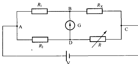
图1 两端式电桥节点位置
